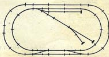
16 rails courbes — 10 rails droits 4 aiguillages droit — 3 aiguillages gauche 13 rails droits de 114 — 3 butoirs
